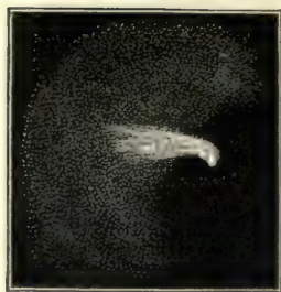
Aug. 18.
